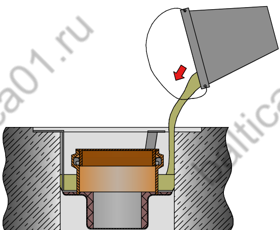
Заполнить пространство строительным раствором нормируемой огнестойкостью
