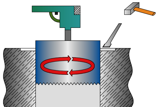
Проделать отверстие в перекрытии
